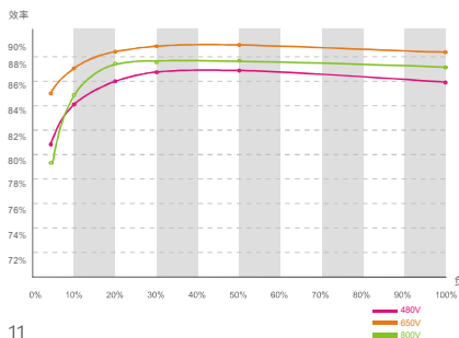
GP 3300 60-160KVA 效率曲线图
